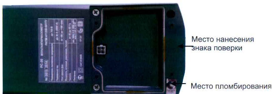
Рисунок 2 – Схема пломбирования
