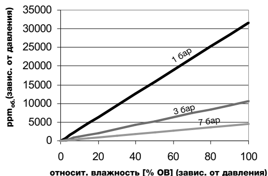
Соотношение относительной влажности и ppm об при 25 °C
