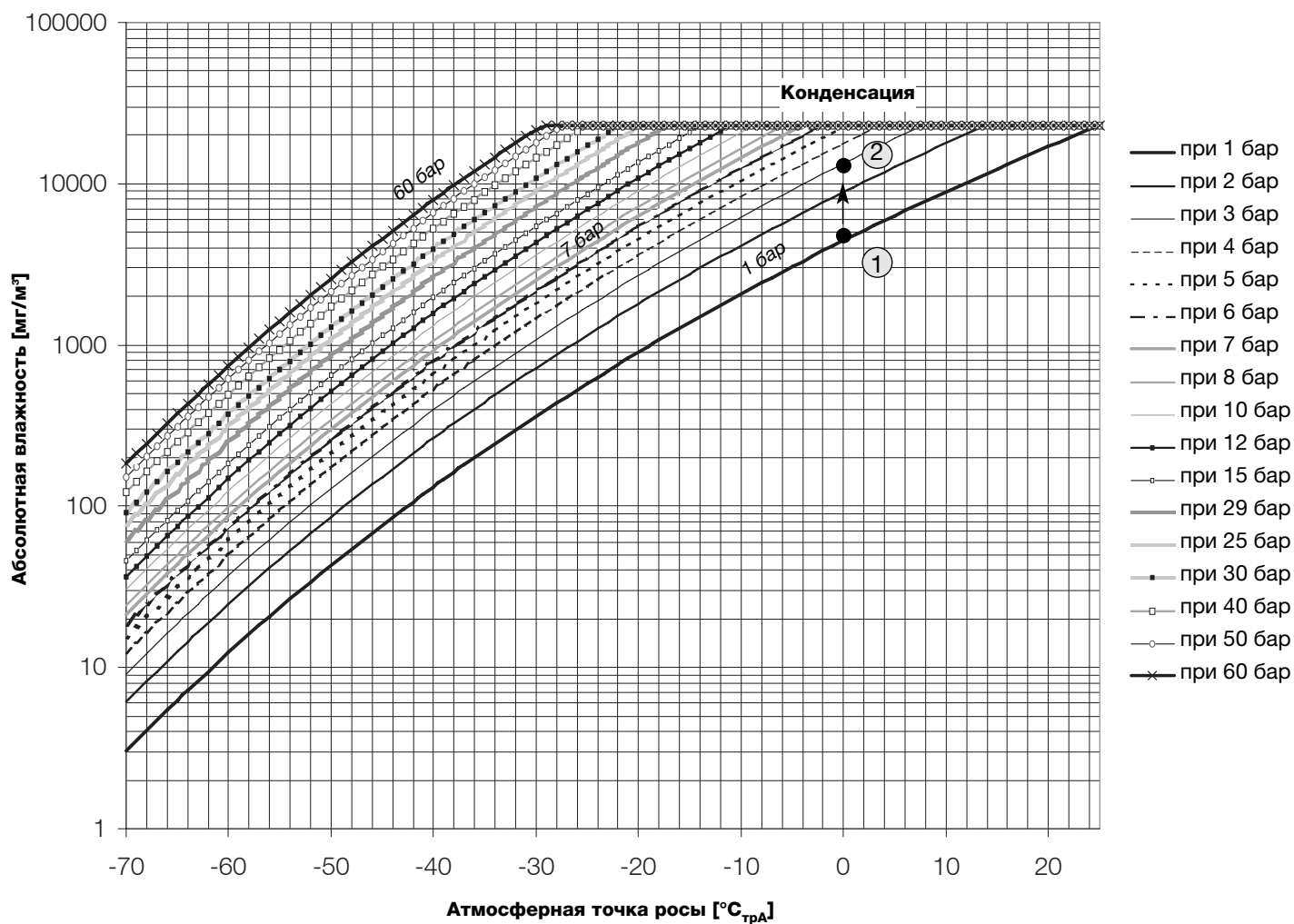
Соотношение атмосферной точки росы и абсолютной влажности при температуре процесса 25 °C
